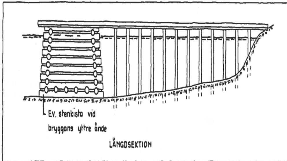
Fig. 2:24 Brygga på stenlista och pålar.
