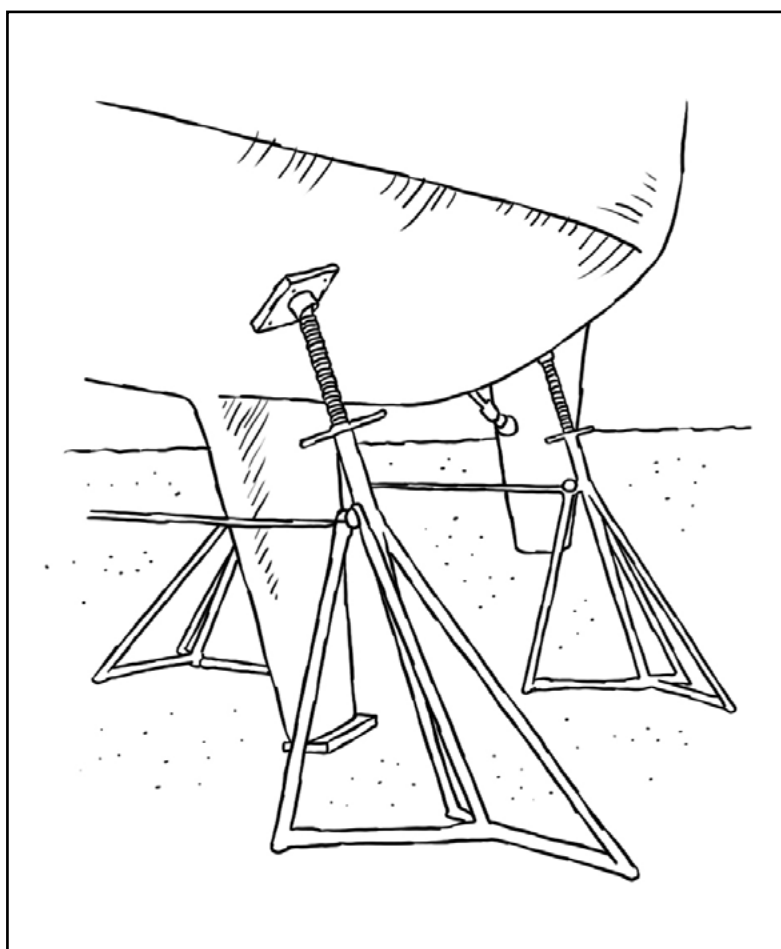
Fig 4:9 Pallning och stötting. Exempel.
