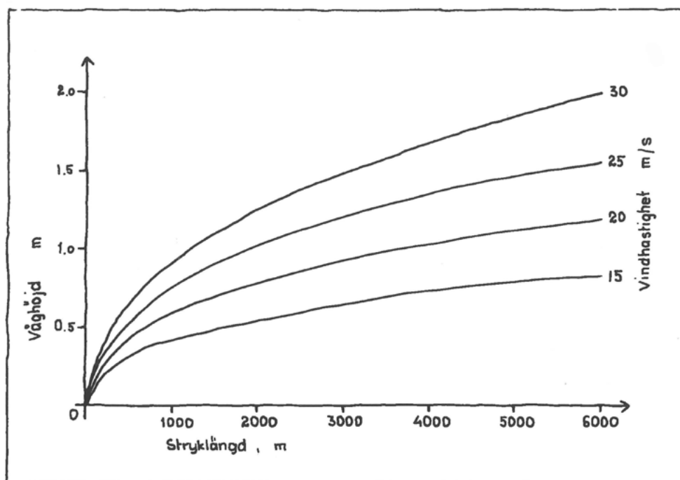
Fig. 2:2 Diagram, våghöjder.
