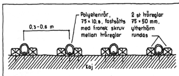
Fig. 4:17 Avvisarverk utfört med plaströr.
