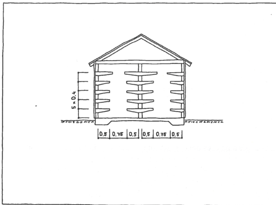
Fig. 4:6 Mastskjul. Sektion.
