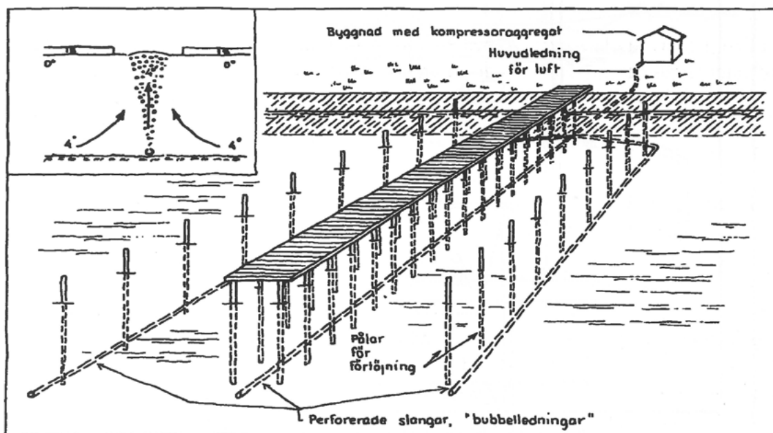
Fig. 2:40 Isbegränsningsanläggning. Luftinblåsning.
