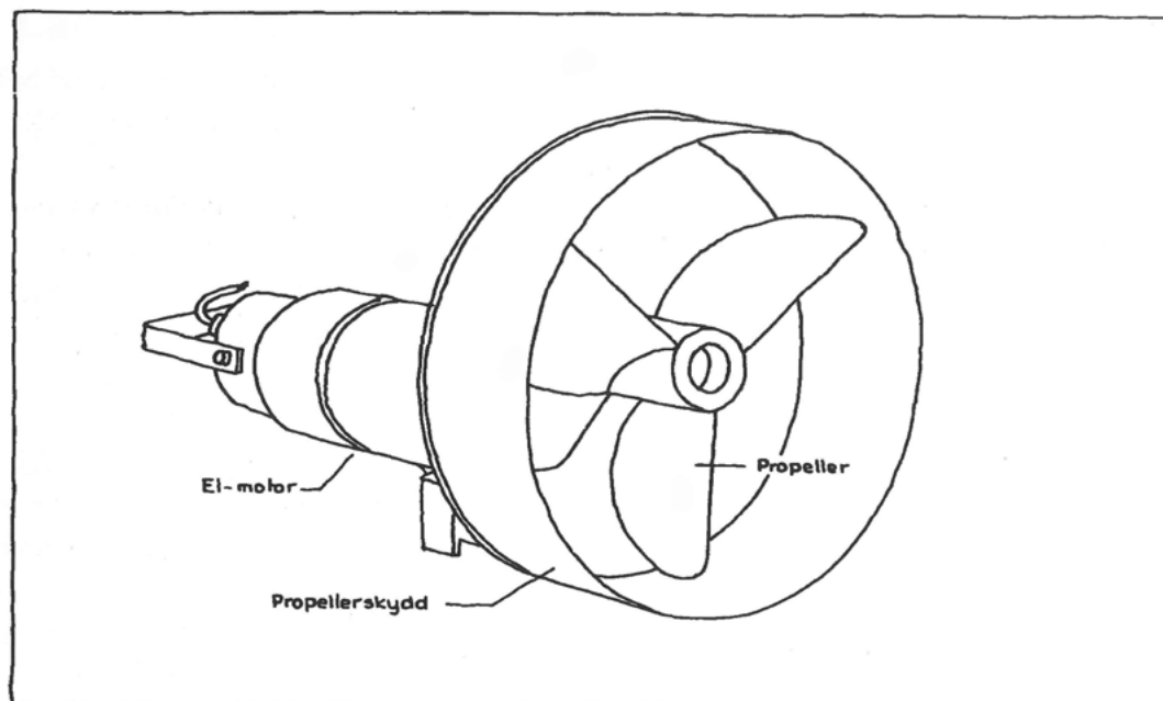
Fig. 2:41 Isbegränsningsanläggning. Strömbildare.
