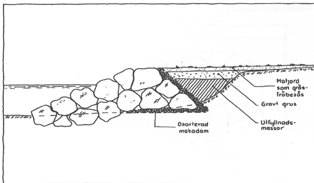
Fig. 4:12 Strandskoning.
