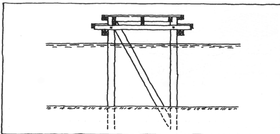
Fig. 2:23 Brygga på pålar. Sektion. Bryggan försedd med längsgående trappsteg.
