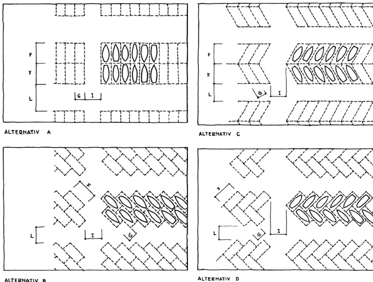
Fig. 4:3 Uppläggningsplatser. Alternativa utformningar. Båtarna placeras utifrån transportmetod.
