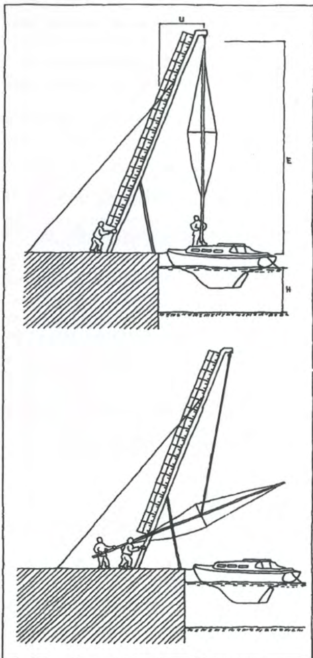
Fig. 3:6 Mastkran.
