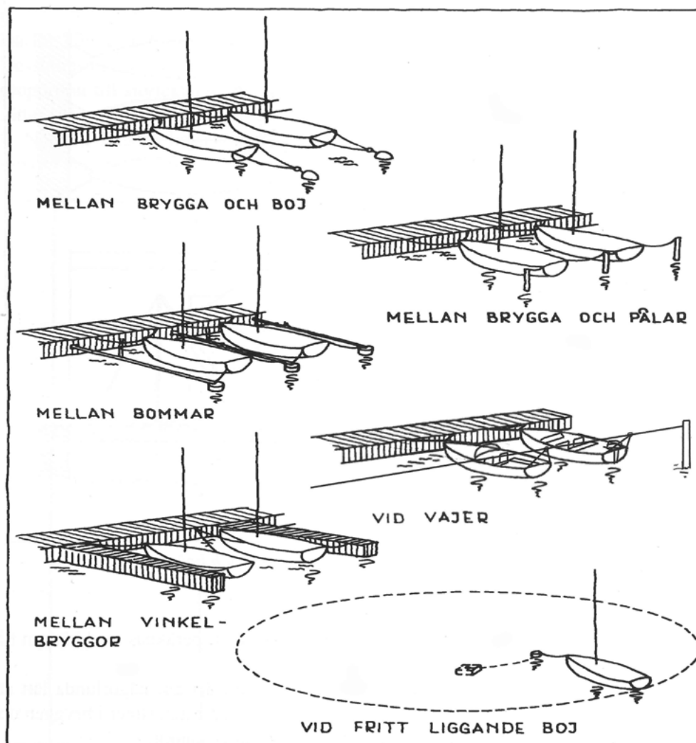
Fig. 2:27 Översikt, förtöjningssätt.
