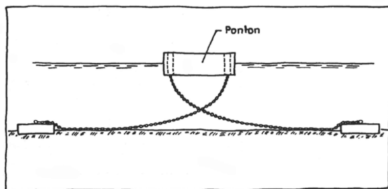
Fig. 2:9.1 Vågbrytande ponton.
