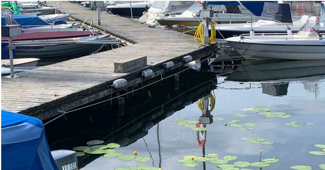
Bild 2:47 Om någon trillar i vattnet kan det vara svårt att nå upp till bryggkant eller båtar. En lina att hålla sig i gör det lättare att ta sig till närmaste räddningsstege, eller in till grunt vatten. Foto: Jimmy Dominus.
