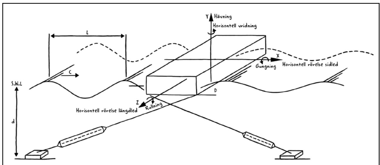
Fig. 2:15 Vågbrytande ponton.
